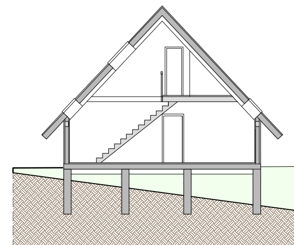
SEZIONE A-A
